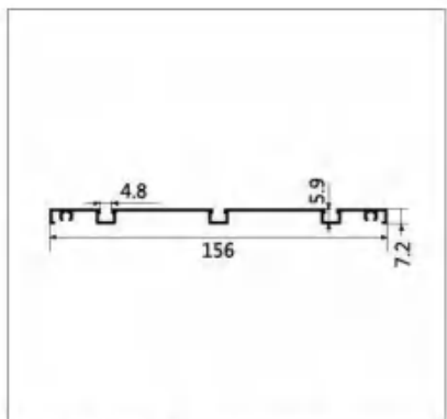
型号:LBW272 名称:三下轨 壁厚:1.3mm 重量:0.851kg/m 长度:6m
