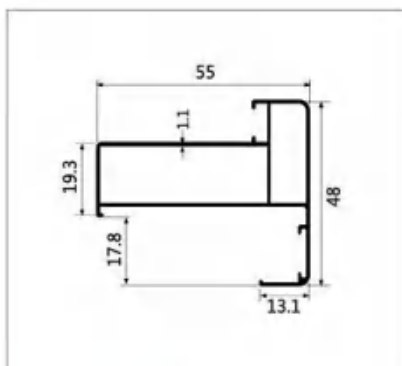
型号:LBW197 名称:1.2 外包 壁厚:1.1mm 重量:0.61kg/m 长度:6.4m
