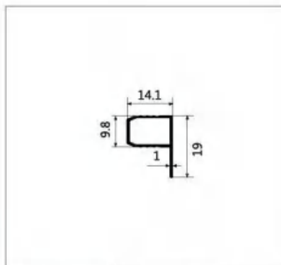
型号:LBW181A 名称:2分P槽 壁厚:1.0mm 重量:0.126kg/m 长度:4.8m
