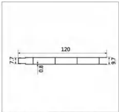
型号:LBW046B 名称:120 扣板 壁厚:0.8mm 重量:0.622kg/m 长度:6.3m
