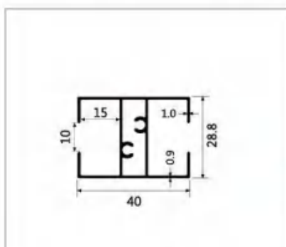
型号:LBW337 名称:单玻光企中柱 壁厚:1.0mm 重量:0.48kg/m 长度:6m
