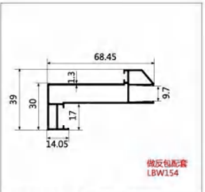
型号:LBW151A 名称:后包框 壁厚:1.3mm 重量:0.801kg/m 长度:6.4m
