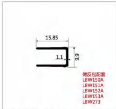
型号:LBW154 名称:反包 F 槽 壁厚:1.1mm 重量:0.113kg/m 长度:6.4m
