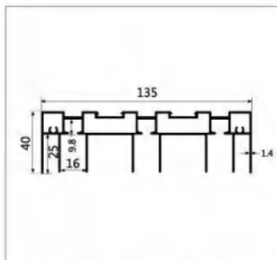
型号:LBW358 名称:三上轨 壁厚:1.4mm 重量:2.286kg/m 长度:6m
