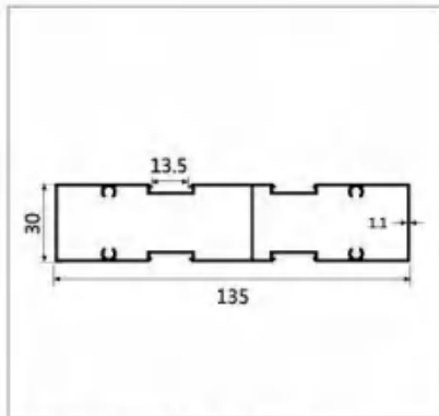
型号:LBW227 名称:三轨中柱 壁厚:1.1mm 重量:1.313kg/m 长度:6m
