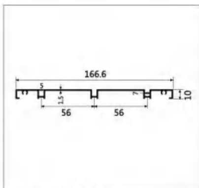
型号:LBW310 名称:三下轨 壁厚:1.5mm 重量:1.04kg/m 长度:6.3m
