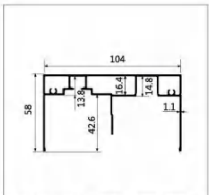
型号:LBW281 名称:2+0联动上轨 壁厚:1.1mm 重量:1.291kg/m 长度:6m
