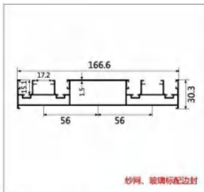
型号:LBW307A 名称:1.6 三边封 壁厚:1.5mm 重量:2.1kg/m 长度:5.6m
