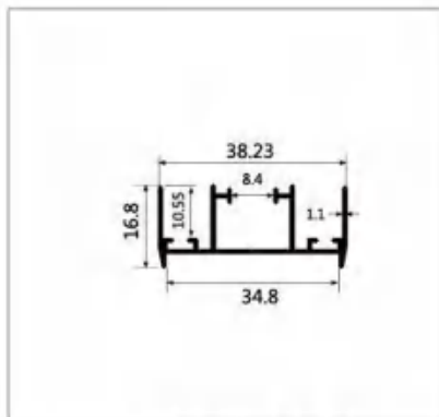
型号:LBW236 名称:推拉收口 壁厚:1.0mm 重量:0.335kg/m 长度:4.8m
