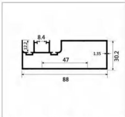
型号:LBW213 名称:1.4 双边封 壁厚:1.35mm 重量:1.031kg/m 长度:4.8m
