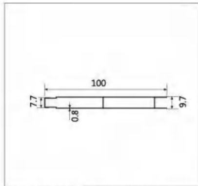
型号:LBW046A 名称:100 扣板 壁厚:0.8mm 重量:0.498kg/m 长度:6.3m
