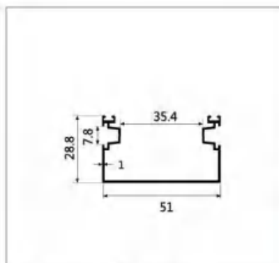
型号:LBW235 名称:双勾企 壁厚:1.0mm 重量:0.38kg/m 长度:4.8m
