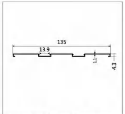
型号:LBW229 名称:三轨中柱盖板 壁厚:1.1mm 重量:0.49kg/m 长度:6m
