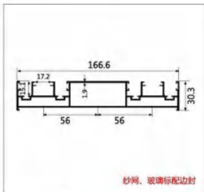
型号:LBW307 名称:2.0 三边封 壁厚:1.9mm 重量:2.4kg/m 长度:5.6m
