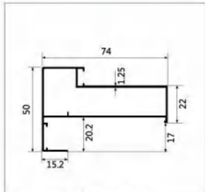
型号:LBW303 名称:正包框 壁厚:1.25mm 重量:0.768kg/m 长度:6.4m
