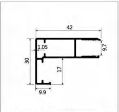
型号:LBW157 名称:前框/包套 壁厚:1.05mm 重量:0.436kg/m 长度:6.4m
