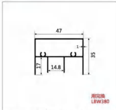
型号:LBW217 名称:单上轨 壁厚:1.0mm 重量:0.57kg/m 长度:6m
