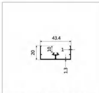
型号:LBW164A 名称:2公分单边封 壁厚:1.0mm 重量:0.34kg/m 长度:4.8m
