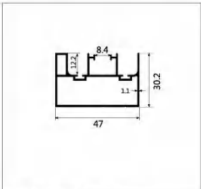
型号:LBW214 名称:单边封 壁厚:1.1mm 重量:0.65kg/m 长度:4.8m
