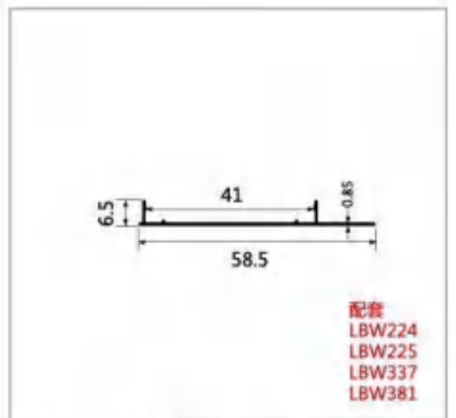
型号:LBW234 名称:吊轨盖板 壁厚:0.85mm 重量:0.164kg/m 长度:6.2m
