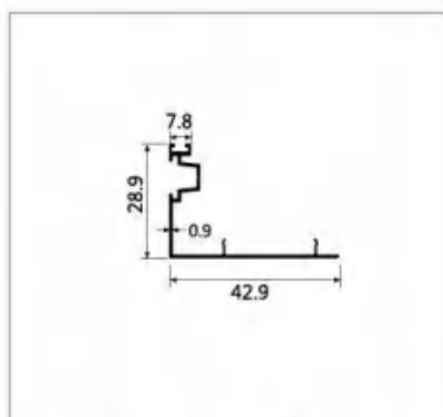
型号:LBW238 名称:单勾企 壁厚:0.9mm 重量:0.237kg/m 长度:4.8m
