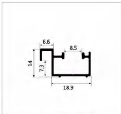
型号:LBW336 名称:纱网料 壁厚:1.0mm 重量:0.18kg/m 长度:6m
