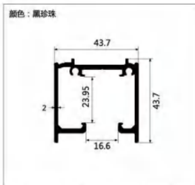
型号:LBW381 名称:单轨吊轨(凹轮) 壁厚:2.0mm 重量:1.006kg/m 长度:5.8m
