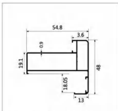
型号:LBW203 名称:1.0 外包 壁厚:0.9mm 重量:0.555kg/m 长度:6.4m
