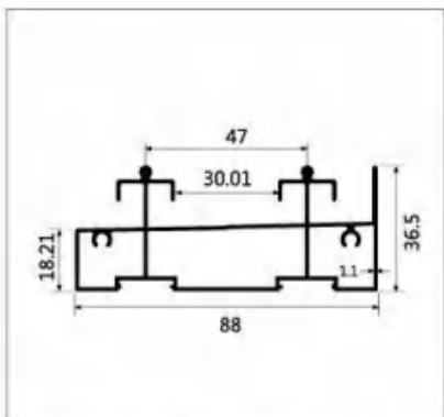
型号:LBW223 名称:两轨高地轨 壁厚:1.1mm 重量:1.223kg/m 长度:6m
