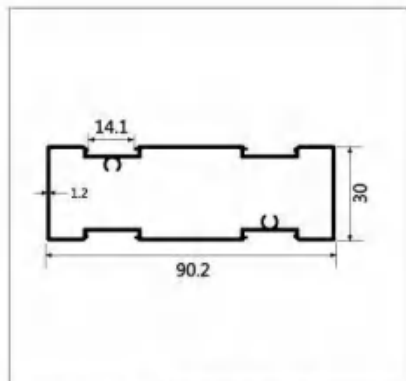
型号:LBW100 名称:两轨中柱 壁厚:1.2mm 重量:0.92kg/m 长度:6m
