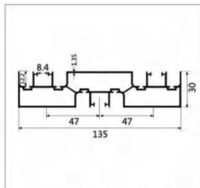
型号:LBW215 名称:1.4 三边封 壁厚:1.35mm 重量:1.855kg/m 长度:5.1m
