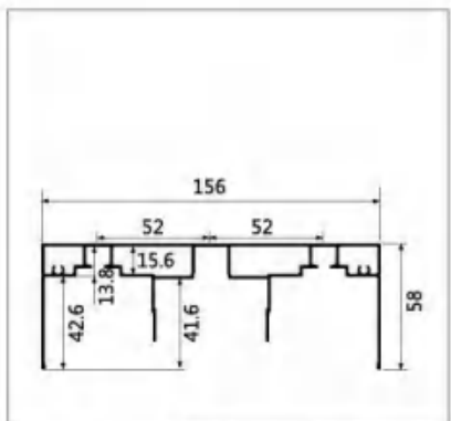
型号:LBW271 名称:推拉三联动上轨 壁厚:1.3mm 重量:2.015kg/m 长度:6m
