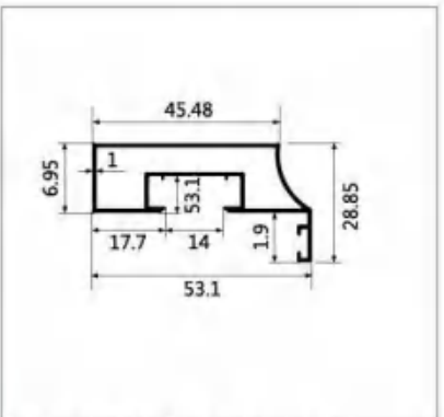
型号:LBW098 名称:平开收口 壁厚:1.0mm 重量:0.496kg/m 长度:4.8m
