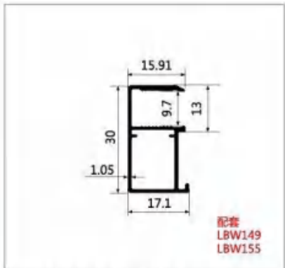
型号:LBW158 名称:包边 壁厚:1.05mm 重量:0.287kg/m 长度:6.4m
