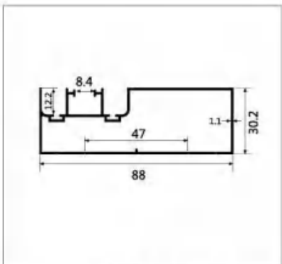
型号:LBW212 名称:1.2 双边封 壁厚:1.1mm 重量:0.87kg/m 长度:4.8m
