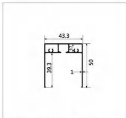
型号:LBW090 名称:单上轨 壁厚:1.0mm 重量:0.587kg/m 长度:6m
