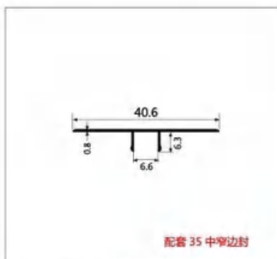
型号:LBW365 名称:35 边封盖板 壁厚:0.8mm 重量:0.11kg/m 长度:5.1m
