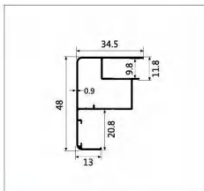
型号:LBW199 名称:前框/包边 壁厚:0.9mm 重量:0.42kg/m 长度:6.4m
