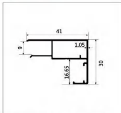
型号:LBW292 名称:前框/包边 壁厚:1.05mm 重量:0.361kg/m 长度:6.4m
