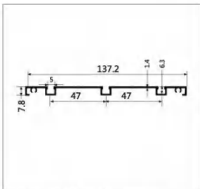
型号:LBW083 名称:三下轨 壁厚:1.4mm 重量:0.791kg/m 长度:6m
