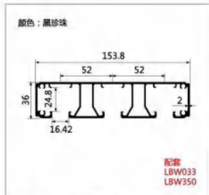
型号:LBW353 名称:三吊轨(凹轮) 壁厚:2.0mm 重量:2.756kg/m 长度:6m
