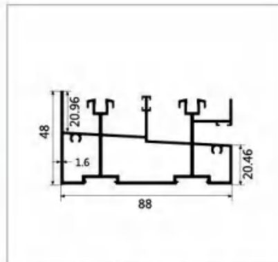
型号:LBW371 名称:两轨高地轨 壁厚:1.6mm 重量:1.846kg/m 长度:6m
