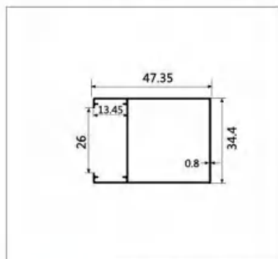
型号:LBW255 名称:0.8 平开光企 壁厚:0.8mm 重量:0.34kg/m 长度:6.2m
