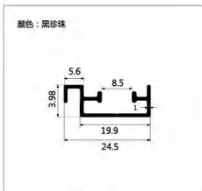
型号:LBW335 名称:纱网料 壁厚:1.0mm 重量:0.165kg/m 长度:6m
