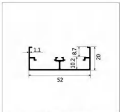
型号:LBW268 名称:单边封 壁厚:1.1mm 重量:0.4kg/m 长度:4.8m
