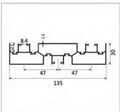
型号:LBW216 名称:1.2 三边封 壁厚:1.1mm 重量:1.56kg/m 长度:5.1m
