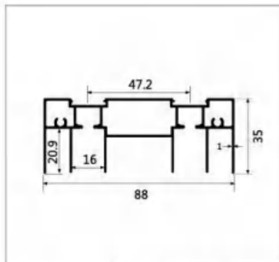
型号:LBW218 名称:双上轨 壁厚:1.1mm 重量:1.2kg/m 长度:6m
