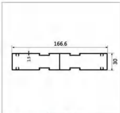
型号:LBW311 名称:三轨中柱 壁厚:1.5mm 重量:1.94kg/m 长度:6.3m
