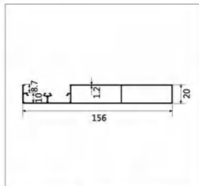
型号:LBW294 名称:三边封 壁厚:1.2mm 重量:1.225kg/m 长度:5.2m
