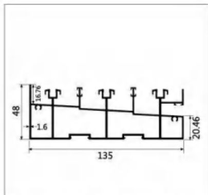
型号:LBW372 名称:三轨高地轨 壁厚:1.6mm 重量:2.623kg/m 长度:6m
