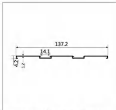
型号:LBW101A 名称:三轨中柱盖板 壁厚:1.2mm 重量:0.533kg/m 长度:6m
