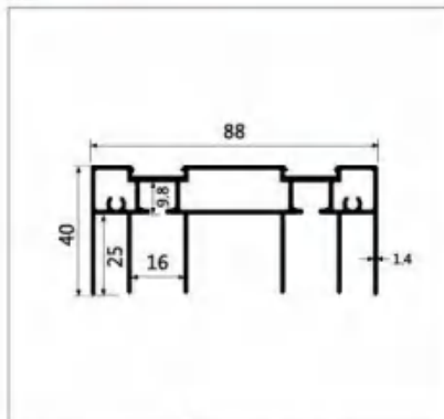
型号:LBW357 名称:双上轨 壁厚:1.4mm 重量:1.614kg/m 长度:6m
