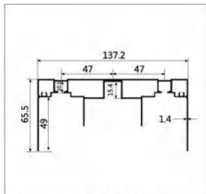
型号:LBW162 名称:三上轨 壁厚:1.4mm 重量:1.782kg/m 长度:6m
