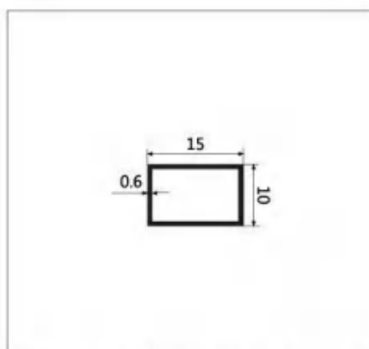
型号:LBW049 名称:10*15格条 壁厚:0.6mm 重量:0.078kg/m 长度:4m
