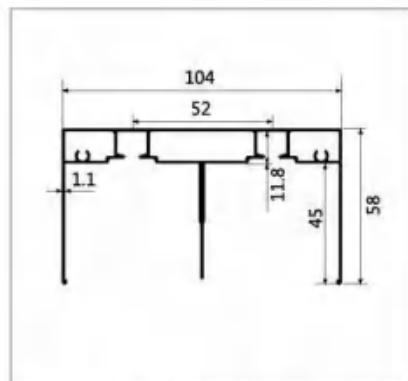
型号:LBW258 名称:推拉双上轨 壁厚:1.1mm 重量:1.326kg/m 长度:6m
