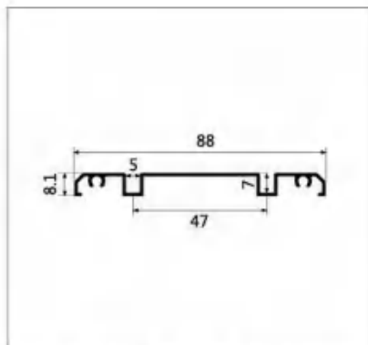
型号:LBW221 名称:双下轨 壁厚:1.1mm 重量:0.45kg/m 长度:6m
