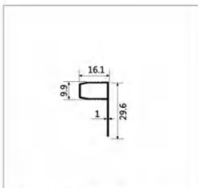
型号:LBW045 名称:三分P槽 壁厚:1.0mm 重量:0.170kg/m 长度:4.8m
