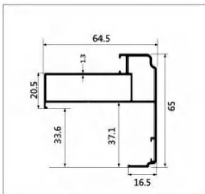
型号:LBW242 名称:1.4 外包 壁厚:1.3mm | 重量:0.86kg/m | 长度:6.4m
