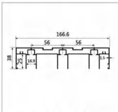
型号:LBW306 名称:三上轨 壁厚:1.5mm 重量:2.37kg/m 长度:6.3m
