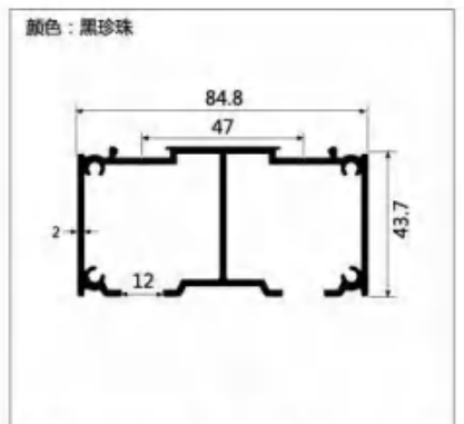
型号:LBW225 名称:双吊轨(平轮) 壁厚:2.0mm 重量:1.65kg/m 长度:6m
