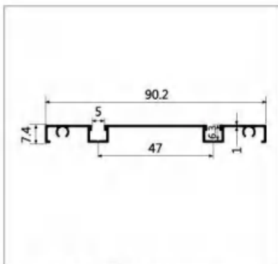
型号:LBW060 名称:双下轨 壁厚:1.0mm 重量:0.416kg/m 长度:6m
