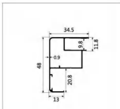
型号:LBW199 名称:前框/包边 壁厚:0.9mm 重量:0.42kg/m 长度:6.4m
