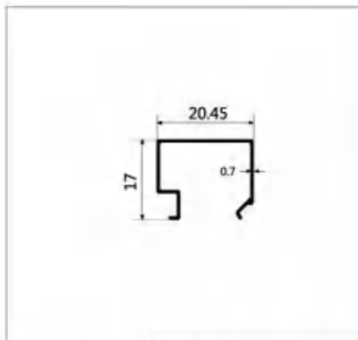
型号:LBW232 名称:方形压线 壁厚:0.7mm 重量:0.12kg/m 长度:6m
