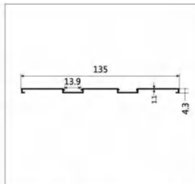
型号:LBW229 名称:三轨中柱盖板 壁厚:1.1mm 重量:0.49kg/m 长度:6m
