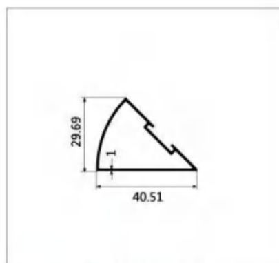
型号:LBW352 名称:转角 壁厚:1.0mm 重量:0.328kg/m 长度:4.8m
