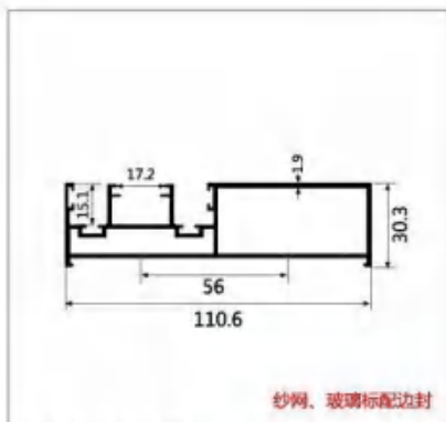
型号:LBW314 名称:2.0 双边封 壁厚:1.9mm 重量:1.6kg/m 长度:5.6m
