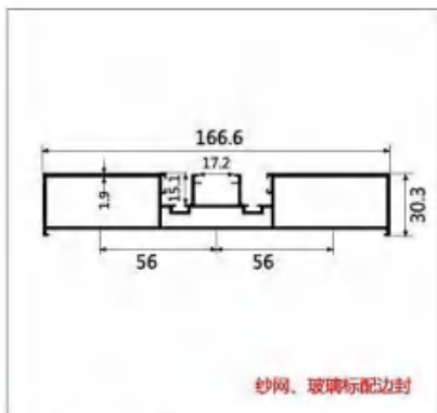
型号:LBW308 名称:2.0 三边封 壁厚:1.9mm 重量:2.24kg/m 长度:5.6m
