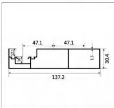
型号:LBW068 名称:三边封 壁厚:1.3mm 重量:1.37kg/m 长度:5.2m
