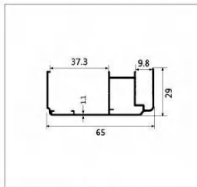
型号:LBW244 名称:前框/包边 壁厚:1.1mm | 重量:0.562kg/m | 长度:6.4m
