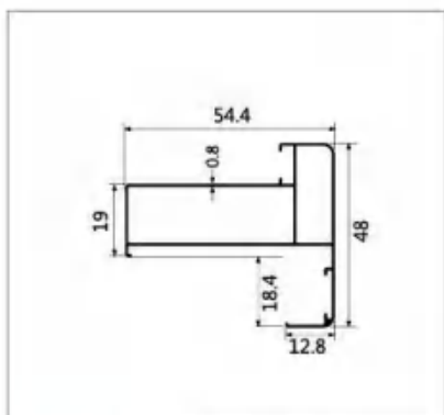
型号:LBW256 名称:0.8 外包 壁厚:0.8mm 重量:0.44kg/m 长度:6.4m
