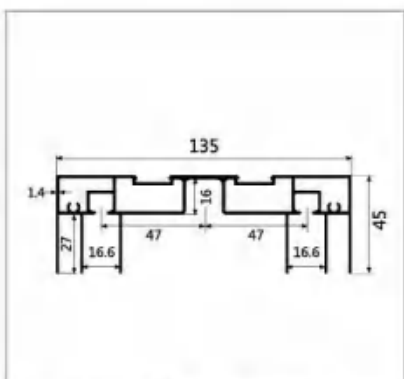
型号:LBW233 名称:三联动上轨 壁厚:1.4 重量:2.11kg/m 长度:6m
