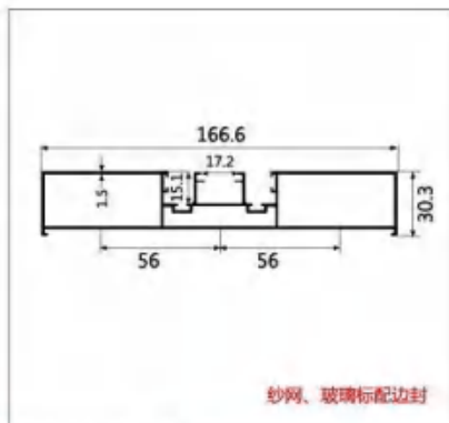
型号:LBW308A 名称:1.6 三边封 壁厚:1.5mm 重量:1.88kg/m 长度:5.6m
