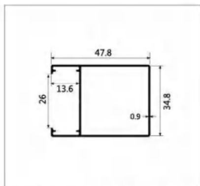
型号:LBW190 名称:1.0 平开光企 壁厚:0.9mm 重量:0.425kg/m 长度:6.2m
