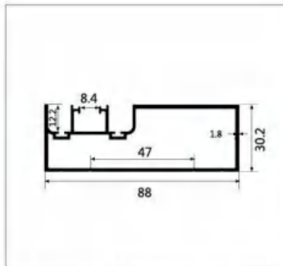
型号:LBW383 名称:2.0 双边封 壁厚:1.8mm 重量:1.2kg/m 长度:4.8m
