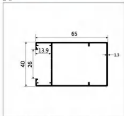
型号:LBW241 名称:1.4 平开光企 壁厚:1.3mm | 重量:0.8kg/m | 长度:5.8m
