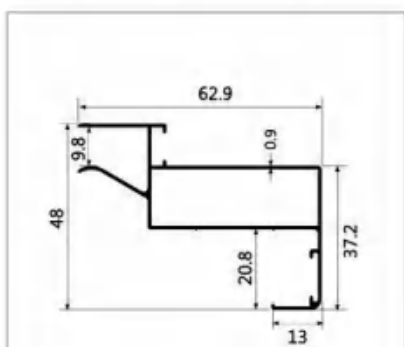
型号:LBW205 名称:1.0 双包后框 壁厚:0.9mm 重量:0.535kg/m 长度:6.4m
