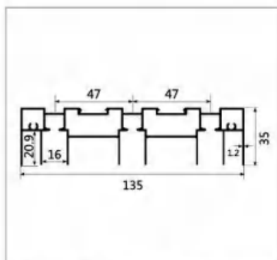
型号:LBW219 名称:三上轨 壁厚:1.2mm 重量:1.8kg/m 长度:6m
