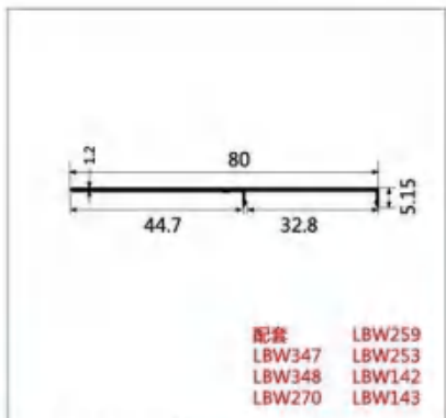
型号:LBW350 名称:凹轮联动吊轨盖板 壁厚:1.2mm 重量:0.281kg/m 长度:6m
