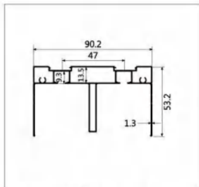
型号:LBW059 名称:双上轨 壁厚:1.0mm 重量:1.186kg/m 长度:6m
