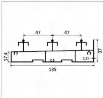
型号:LBW230 名称:三轨高地轨 壁厚:1.25mm 重量:1.74kg/m 长度:6m
