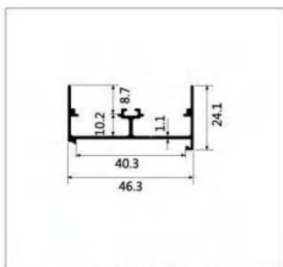
型号:LBW266 名称:推拉收口 壁厚:1.1mm 重量:0.386kg/m 长度:4.8m
