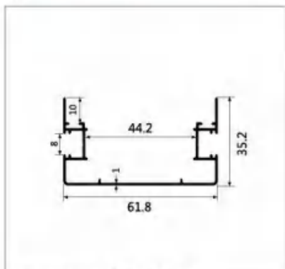
型号:LBW330 名称:双勾企 壁厚:1.0mm 重量:0.52kg/m 长度:5.2m
