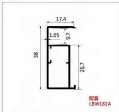
型号:LBW158A 名称:包边 壁厚:1.05mm 重量:0.32kg/m 长度:6.4m
