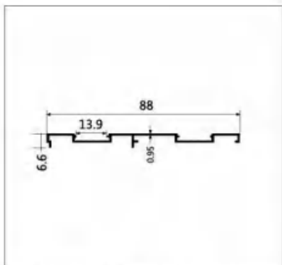
型号:LBW228 名称:两轨中柱盖板 壁厚:0.95mm 重量:0.33kg/m 长度:6m
