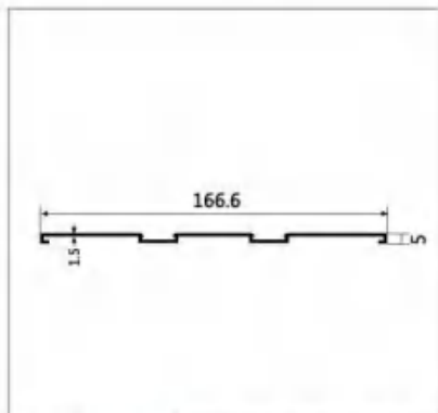
型号:LBW312 名称:三轨中柱盖板 壁厚:1.5mm 重量:0.8kg/m 长度:6.3m
