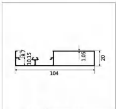
型号:LBW257 名称:双边封 壁厚:1.05mm 重量:0.759kg/m 长度:4.8m
