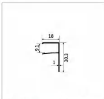
型号:LBW079 名称:三分F槽 壁厚:1.0mm 重量:0.165kg/m 长度:6.2m
