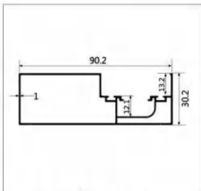
型号:LBW061 名称:双边封 壁厚:1.0mm 重量:0.791kg/m 长度:4.8m
