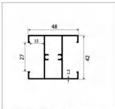
型号:LBW323 名称:中柱 壁厚:1.2mm 重量:0.722kg/m 长度:6.3m
