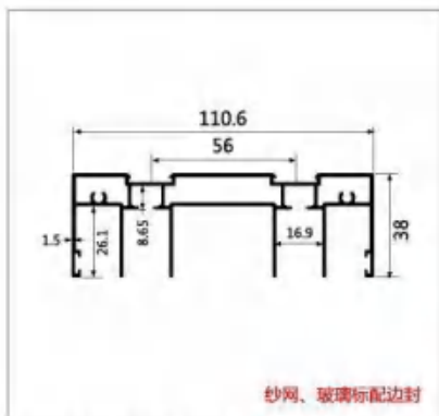
型号:LBW313 名称:双上轨 壁厚:1.5mm 重量:1.62kg/m 长度:6.3m
