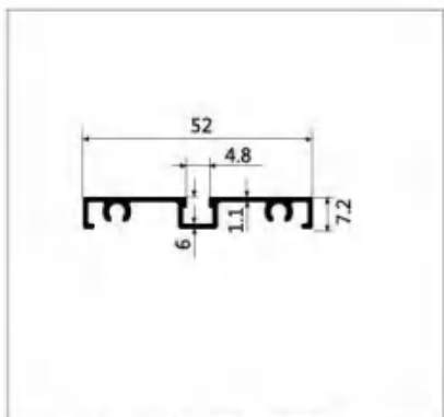
型号:LBW267 名称:单下轨 壁厚:1.1mm 重量:0.34kg/m 长度:6m
