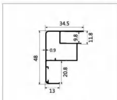
型号:LBW199 名称:前框/包边 壁厚:0.9mm 重量:0.42kg/m 长度:6.4m
