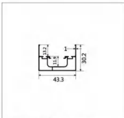
型号:LBW092 名称:单边封 壁厚:1.0mm 重量:0.48kg/m 长度:4.8m
