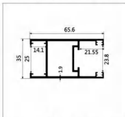
型号:LBW250 名称:2.0 推拉光企 壁厚:1.9mm 重量:1.1kg/m 长度:6.3m
