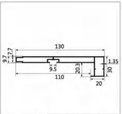
型号:LBW175 名称:130 加长包套 壁厚:1.35mm 重量:1.276kg/m 长度:6.4m
