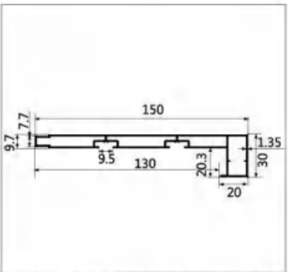
型号:LBW177 名称:150 加长包套 壁厚:1.35mm 重量:1.49kg/m 长度:6.4m
