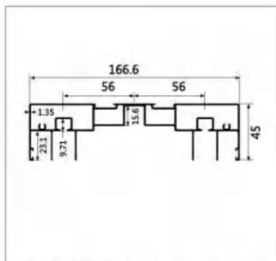
型号:LBW351 名称:三联上轨 壁厚:1.35mm 重量:2.435kg/m 长度:6.3m
