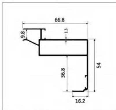
型号:LBW243 名称:1.4 后框 壁厚:1.3mm | 重量:0.78kg/m | 长度:6.4m
