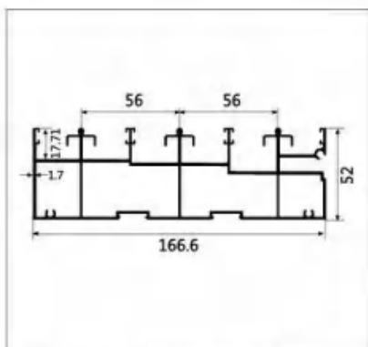
型号:LBW309 名称:三轨高地轨 壁厚:1.7mm 重量:3.3kg/m 长度:6.3m
