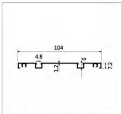
型号:LBW295 名称:双下轨 壁厚:1.2mm 重量:0.575kg/m 长度:6m
