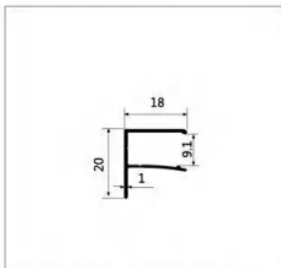
型号:LBW137 名称:2分F槽 壁厚:1.0mm 重量:0.14kg/m 长度:6.2m
