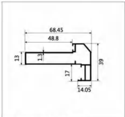
型号:LBW150A 名称:正包 壁厚:1.3mm 重量:0.75kg/m 长度:6.4m
