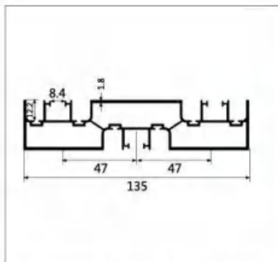
型号:LBW384 名称:2.0 三边封 壁厚:1.8mm 重量:2.12kg/m 长度:5.1m
