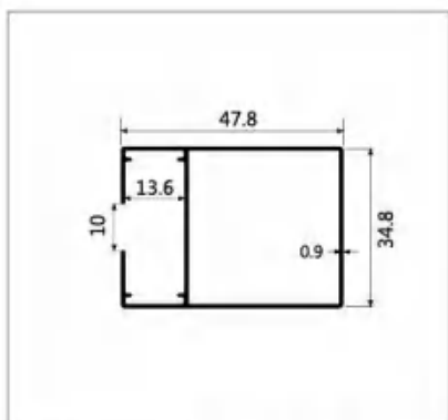
型号:LBW325 名称:1.0 平开单玻光企 壁厚:0.9mm 重量:0.47kg/m 长度:6.2m
