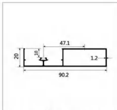
型号:LBW163A 名称:2公分双边封 壁厚:1.2mm 重量:0.7kg/m 长度:4.8m
