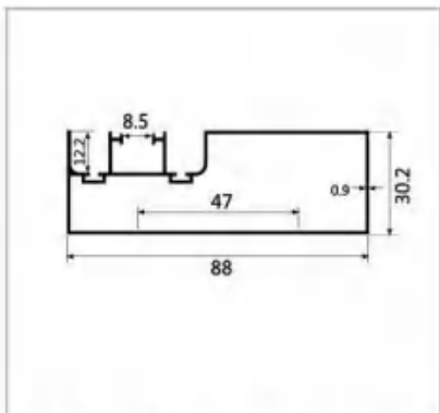
型号:LBW211 名称:1.0 双边封 壁厚:0.9mm 重量:0.74kg/m 长度:4.8m
