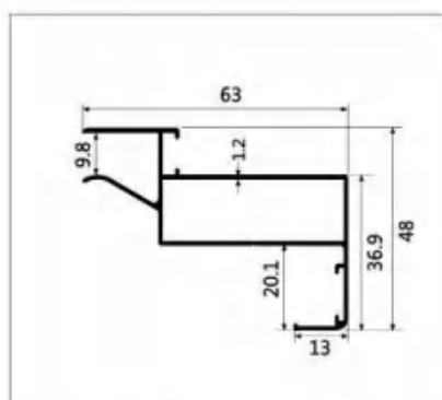
型号:LBW200 名称:1.2 双包后框 壁厚:1.2mm 重量:0.63kg/m 长度:6.4m
