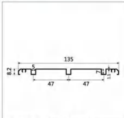
型号:LBW222 名称:三下轨 壁厚:1.1mm 重量:0.64kg/m 长度:6m
