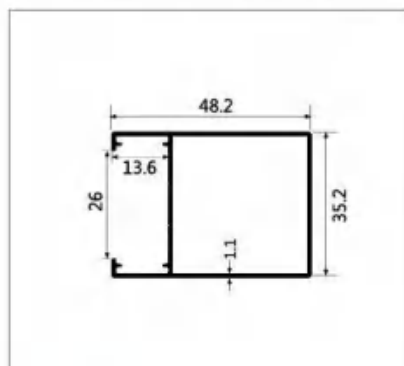
型号:LBW191 名称:1.2 平开光企 壁厚:1.1mm 重量:0.527kg/m 长度:6.2m
