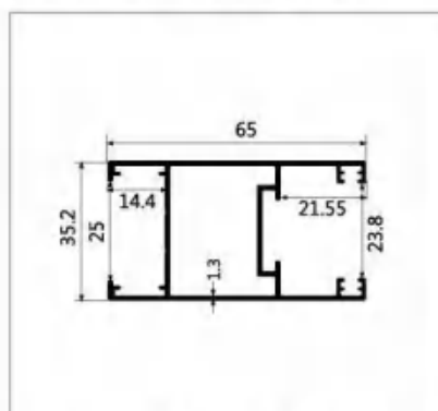
型号:LBW249 名称:1.4 推拉光企 壁厚:1.3mm 重量:0.86kg/m 长度:6.3m
