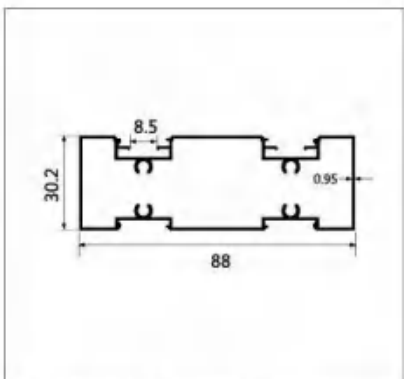
型号:LBW226 名称:两轨中柱 壁厚:0.95mm 重量:0.91kg/m 长度:6m
