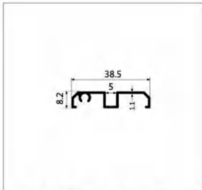
型号:LBW220 名称:单下轨 壁厚:1.2mm 重量:0.244kg/m 长度:6m
