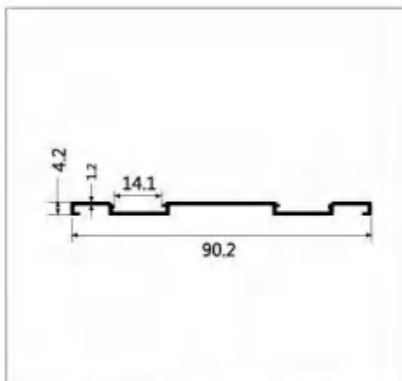
型号:LBW100A 名称:两轨中柱盖板 壁厚:1.2mm 重量:0.376kg/m 长度:6m
