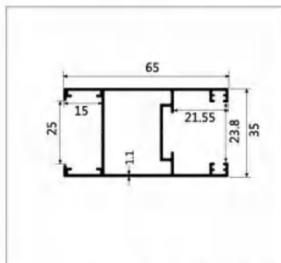
型号:LBW248 名称:1.2 推拉光企 壁厚:1.1mm 重量:0.754kg/m 长度:6.3m
