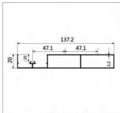
型号:LBW165A 名称:2公分三边封 壁厚:1.2mm 重量:1.063kg/m 长度:5.2m
