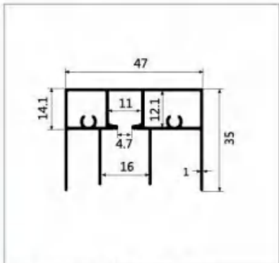
型号:LBW380 名称:单上轨 壁厚:1.0mm 重量:0.66kg/m 长度:5.8m
