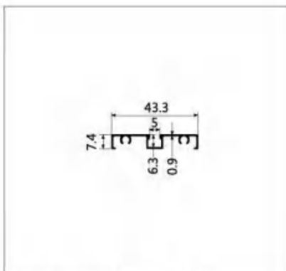
型号:LBW091 名称:单下轨 壁厚:0.9mm 重量:0.233kg/m 长度:6m
