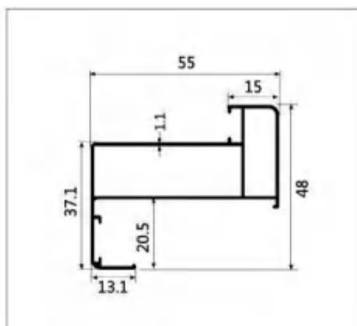
型号:LBW198 名称:1.2 内包 壁厚:1.1mm 重量:0.61kg/m 长度:6.4m
