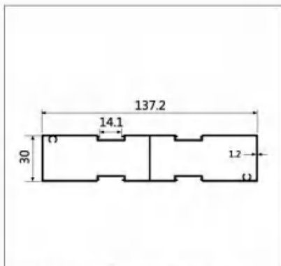
型号:LBW101 名称:三轨中柱 壁厚:1.2mm 重量:1.31kg/m 长度:6m
