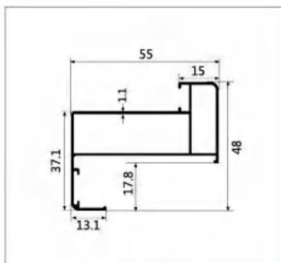
型号:LBW198 名称:1.2 内包 壁厚:1.1mm 重量:0.61kg/m 长度:6.4m
