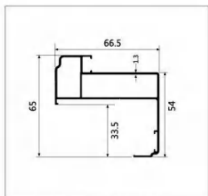
型号:LBW305 名称:1.4 内包 壁厚:1.3mm | 重量:0.855kg/m | 长度:6.4m
